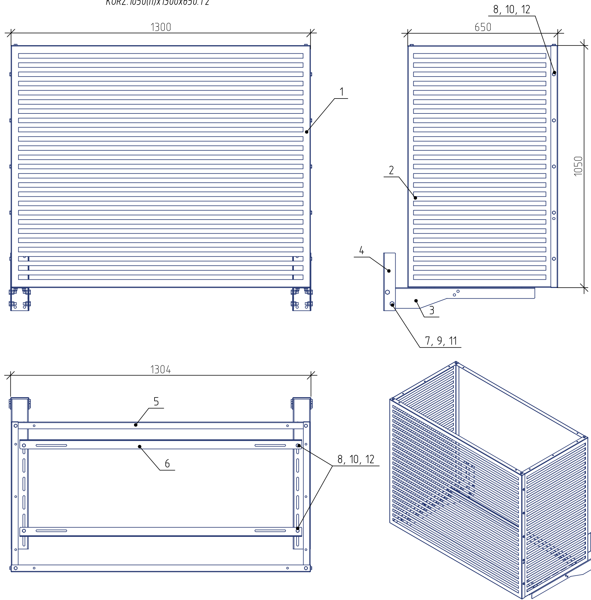
Корзина для кондиционера KORZ.1050(h)x1300x650.T2
